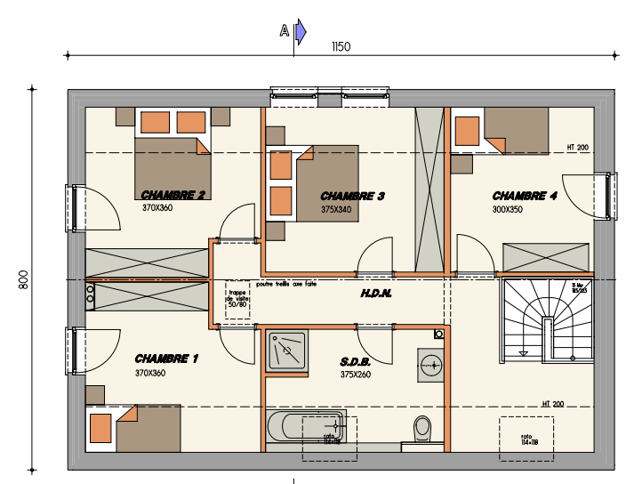
ETAGE
