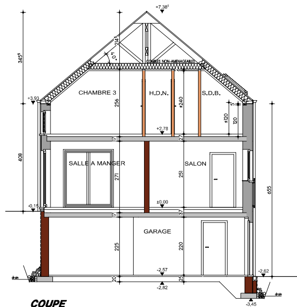
COUPE
