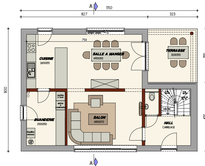
REZ-DE-CHAUSSEE
