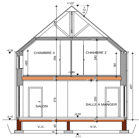
COUPE
