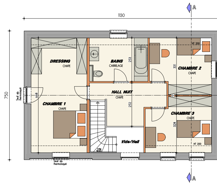
ETAGE
