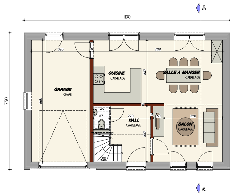
REZ-DE-CHAUSSEE
